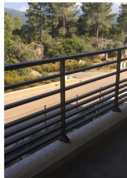
LOIG Garde-corps. Pose sur dalle. Main courante rectangle KAY. Coloris Gris Anthracite - RAL 7016
